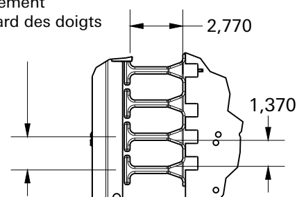
DÉTAIL A (ESPACEMENT DES DOIGTS)
