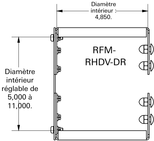
Vue de dessus Anneau D simple
