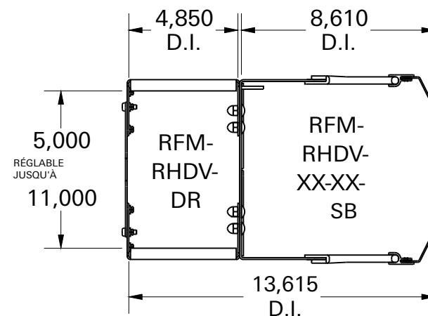
VUE DE DESSUS ANNEAU EN D ASSEMBLÉ SUR RHDV-SB
