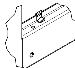
DÉTAIL C INSTALLER AVANT PEINTURE
