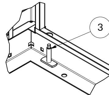
DÉTAIL B INSTALLER APRÈS PEINTURE
