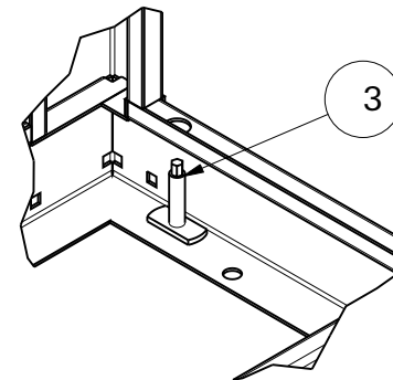
DÉTAIL A À installer après peinture
