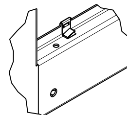
DÉTAIL C À installer avant peinture
