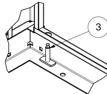
DÉTAIL B À installer après peinture
