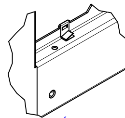
DÉTAIL C À INSTALLER AVANT PEINTURE
