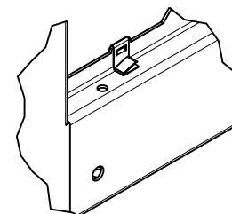
DÉTAIL C À INSTALLER AVANT PEINTURE
