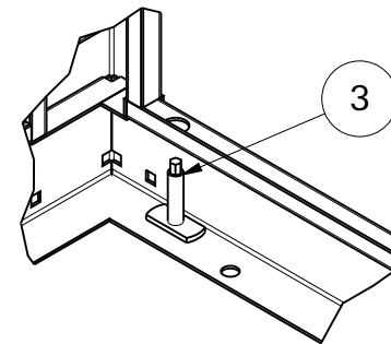
DÉTAIL B À INSTALLER APRÈS PEINTURE
