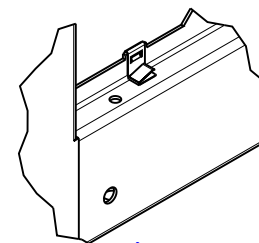
DÉTAIL C À INSTALLER AVANT PEINTURE
