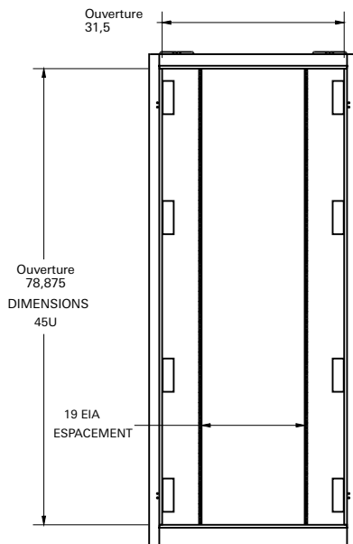
AVANT PORTE RETIRÉE
