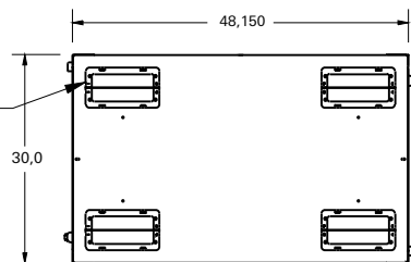
HAUT
